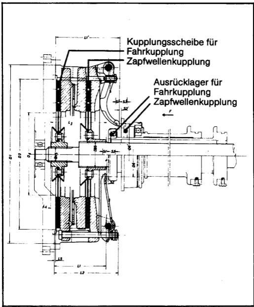
Abb. 461 Schemazeichnung einer Zweifachkupplung S_2 = Kupplungsspiel
